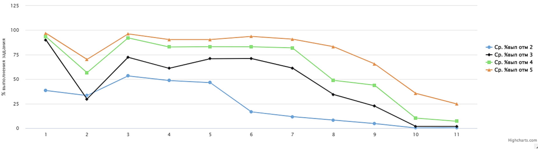
ВПР 2024 / 8 Физика
